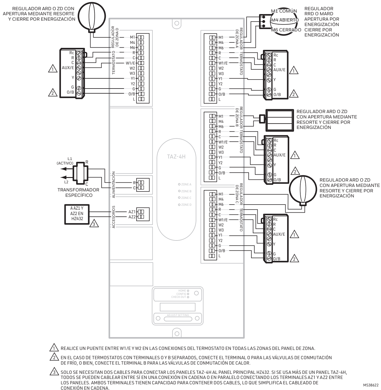
Fig. 8. Cableado del panel de zona de la bomba de calor de 2 etapas de calor y 1 etapa de frío, con calor auxiliar eléctrico.
