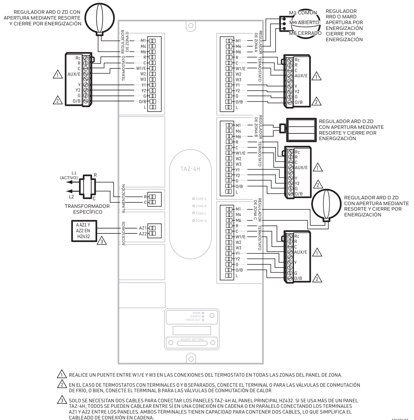
Fig. 9. Cableado del panel de zona con la bomba de calor, 3 etapas de calor y 2 etapas de frío, con 3 etapas de calor eléctrico.
