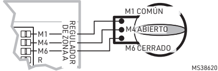
Fig. 6. Cableado del regulador.
