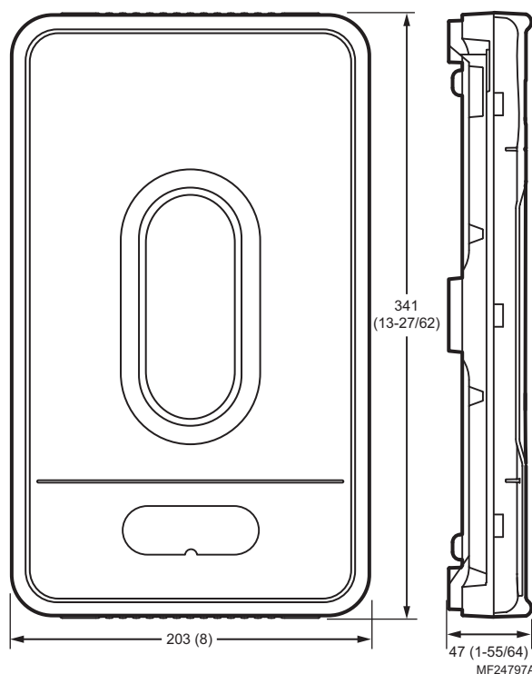
Fig. 1. Dimensions du panneau de zone TAZ-4H en millimètres (pouces).
