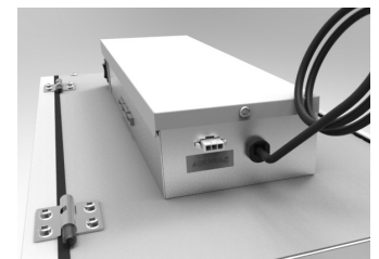
Figure 1 * Connecteur auxiliaire pour câblage de volet externe. Non-inclus: harnais de câblage et moteur de volet.
