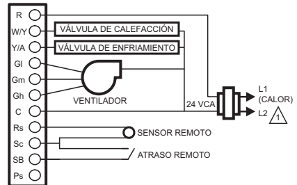
Fig. 15. Diagrama de cableado de dos tubos (calefacción o enfriamiento) con relevo automático (24 VCA en la ilustración).
