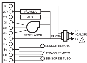
Fig. 18. Diagrama de cableado de cuatro tubos (calefacción y enfriamiento) con relevo manual/automático (24 VCA en la ilustración).
