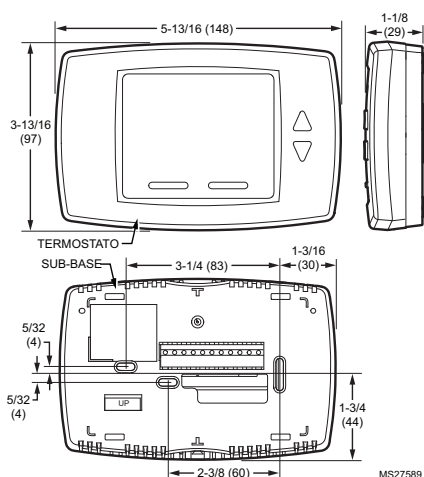
Fig. 1. Dimensiones en pulgadas (milímetros).
