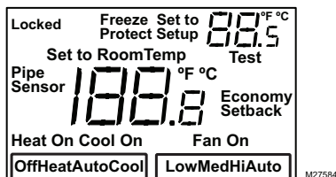
Fig. 22. Pantalla LCD con todos los elementos que pueden aparecer.
