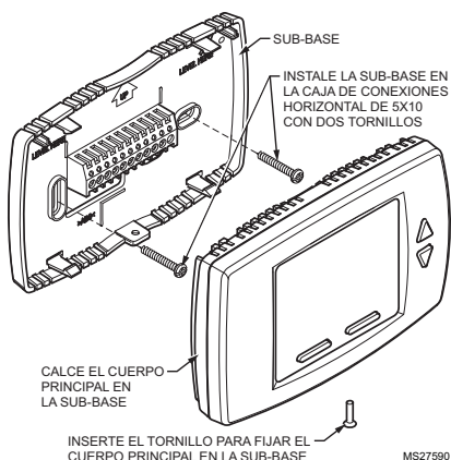
Fig. 2. Instalación de la subbase y el termostato en una caja de conexiones de 5 x 10 cm (2 x 4 pulg.).
