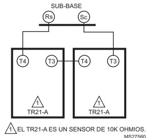
Fig. 5. Cableado de dos sensores TR21-A (10K ohmios) para proporcionar una red de determinación promedio de la temperatura.
