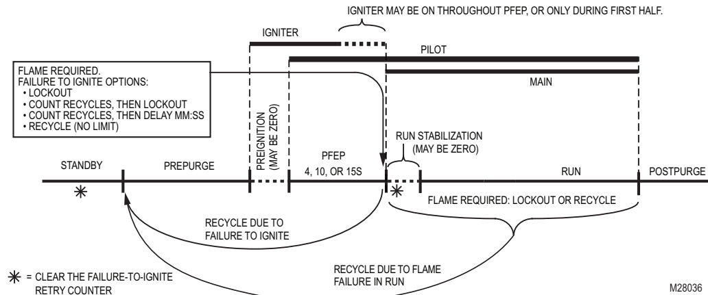
Fig. 24. Intermittent pilot.
