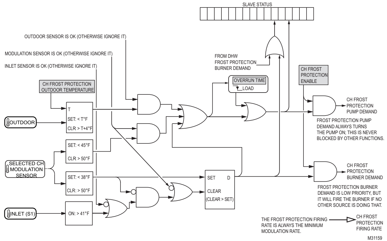
Fig. 17. CH Frost protection.
