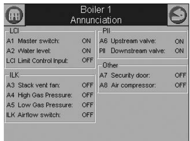
Fig. 27. Annunciator display.
