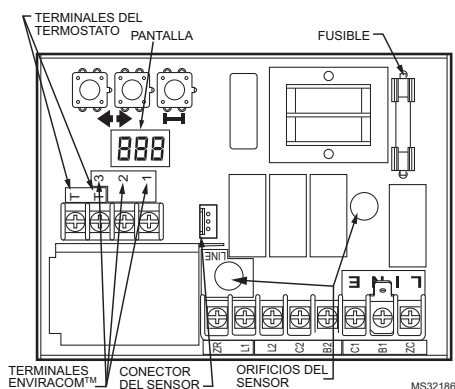
Fig. 3. Circuito impreso con las conexiones del sensor y los orificios del cilindro para los modelos de montaje horizontal.
