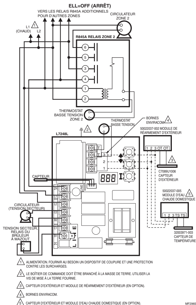
Fig. 11. L7228L système multizones avec connexions du circulateur.
