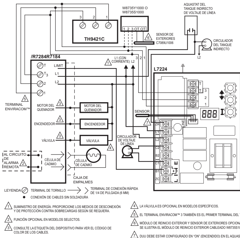
Fig. 10. L7224A,C; L7248L con sistema de una zona con circulador y tanque de agua indirecto con termostato EnviraCOM™.
