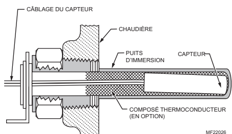
Fig. 4. Installation du capteur de rechange.
