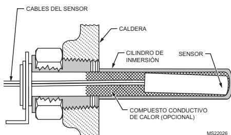
Fig. 4. Instalación del sensor de reemplazo.
