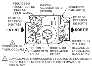
Fig. 1. Vue dessus de l'appareil de contrôle du gaz de la combinaison VR8200.
