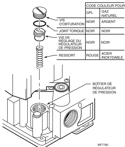
Fig. 2. Installation de la trousses de conversion dans le régulateur.
