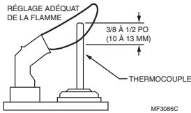
Fig. 3. Réglage approprié de la flamme.
