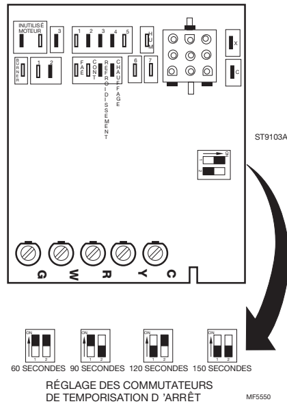
Fig. 3. Réglage des commutateurs de temporisation d'arrêt.
