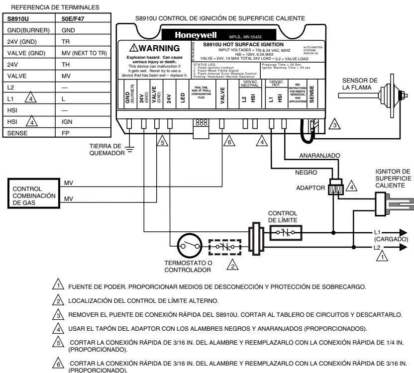
La Fig. 3. Instalación típico cuando el S8910U reemplaza el 50E/F47 de White-Rodgers.
