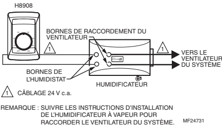
Fig. 16. Raccordement du H8908 avec un humidificateur à vapeur.
