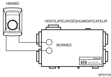
Fig. 18. Schéma de raccordement typique dans des applications de ventilation avec un HR150, HR200, ER150 et ER200 ou de déshumidification avec un DH90.
