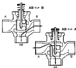
Fig. 1. Inwendige doorstroming bij drieweg verdeelafsluiters.
