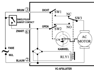
Fig. 6. Motorbesturing Serie 80 met enkelpolig aan/uit schakelcontact
