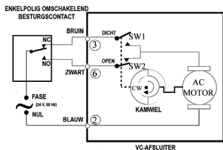
Fig. 5. Motorbesturing Serie 20 met enkelpolig omschakelcontact.
