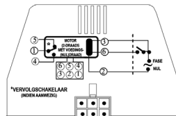
Fig. 3. Bedravingsvoorbeeld Serie 20 voor besturing met enkelpolig omschakecontact.
