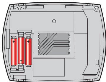
Parte posterior del termostato.
