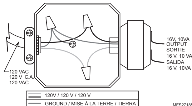
FIG. 1: LINE VOLT CONNECTION RACCORDEMENT AU SECTEUR CONEXIÓN AL SUMINISTRO DE TENSIÓN DE LÍNEA
